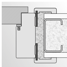
montáž do pěny do stěny ze sádrokartonové desky
