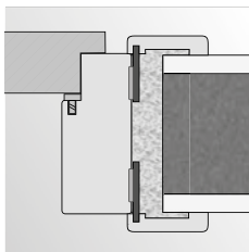
montáž do pěny do zděné stěnyj
