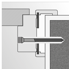
montáž do pěny a kotvy do zděné stěny
