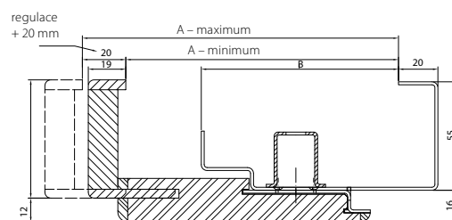
PRŮŘEZ ZÁRUBNĚ PROJEKT Premium
