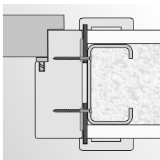
montáž na vruty do stěny ze sádrokartonové desky
