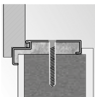
rohová zárubeň velká montáž pomocí hmoždinek
