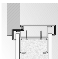
rohová zárubeň velká montáž do sádrokartonové stěny
