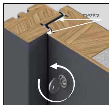
PO zavření ~ 3 mm
