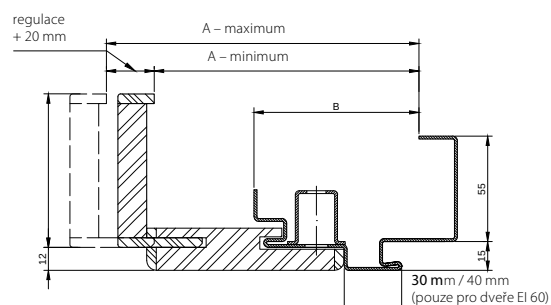
PRŮŘEZ ZÁRUBNĚ PROJEKT
