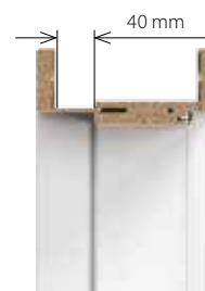
maximální zárubeň s širokým perem volitelně za příplatek
