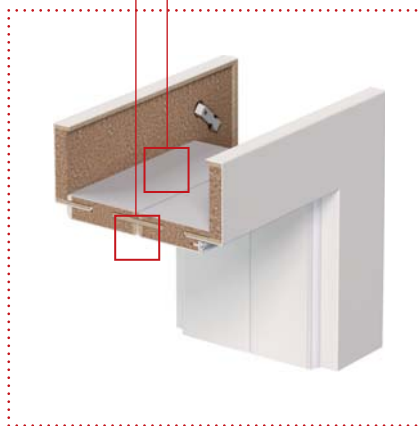
ŘEZ SLOŽENÉ ZÁRUBNĚ / REZ ZLOŽENEJ ZÁRUBNE
