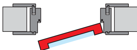
ZPŮSOB MONTÁŽE MATNÉHO SKLA (KŘÍDLO PRAVÉ – MATNÁ ČÁST SMĚREM K POZORUJÍCÍMU) /
