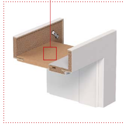
ŘEZ ZÁRUBNĚ S REGULAČNÍM PANELEM / REZ ZÁRUBNE S REGULAČNÝM PANELEM
