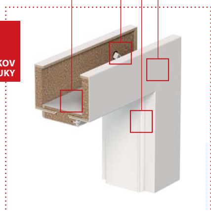
ŘEZ ZÁKLADNÍ ZÁRUBNĚ / REZ ZÁKLADNEJ ZÁRUBNE
